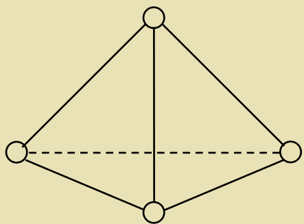
图11 正四面体
