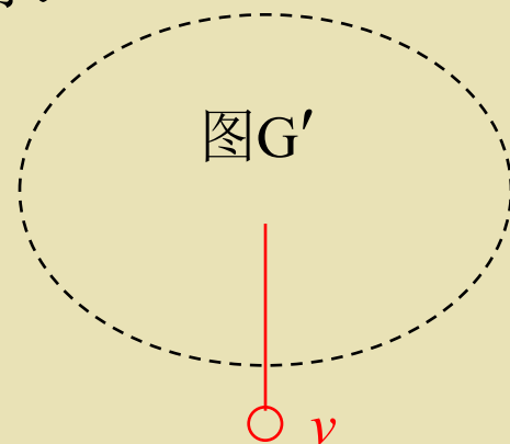
图9.图G
