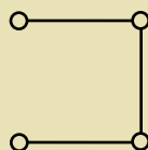
图13. 图 G 的闭包
