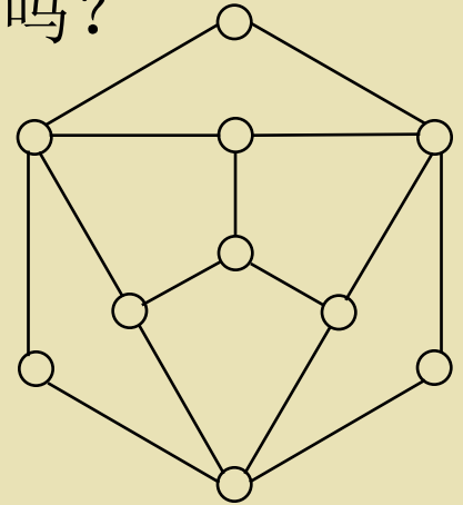
图8. G
