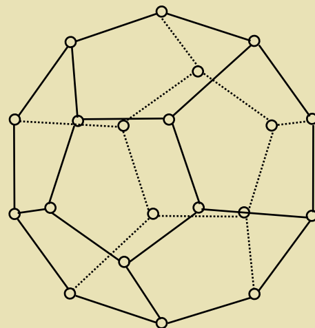
图13 正十二面体
