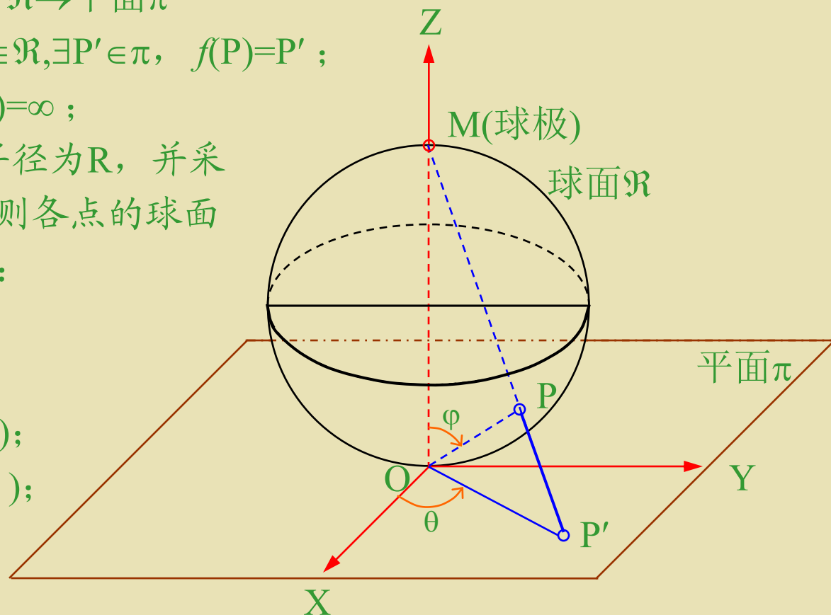
图14. 球极平面投影
