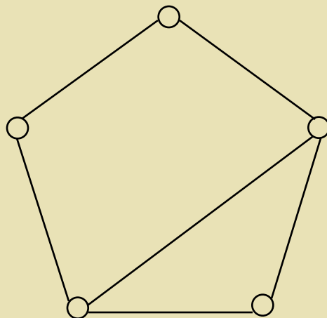
(a) 图 G_2
